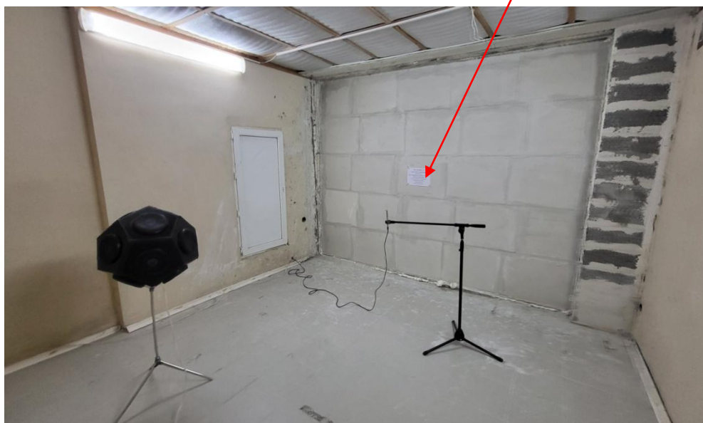
Фото 1. Камера высокого уровня, испытание фрагмента перегородки из плит гипсовых пазогребневых полнотелых ПлГН1 667x500x80 выложенных на монтажном гипсовом клее «ПЕРЛГИПС», толщина перегородки 80 мм Регистрационный № 4981-25 в акустической камере
