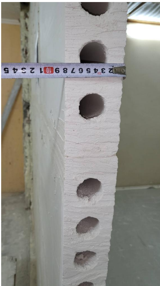
Фото 1. Изготовление фрагмента перегородки в акустической камере, (плиты гипсовые пазогребневые пустотелые ПЛГН2 размером 667x500x80)
